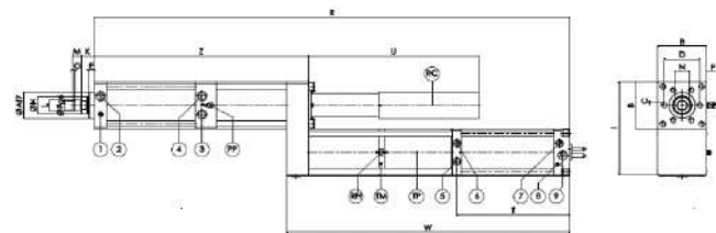
Abbildung 1.1 _ Schematische Ansicht der Einheit VERSION „NG“
