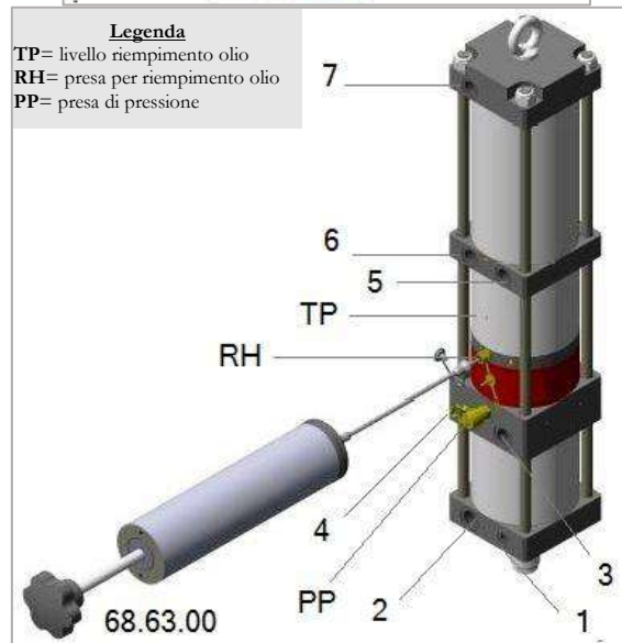
Figura 6 - Collegamento pompa di ricarica olio
