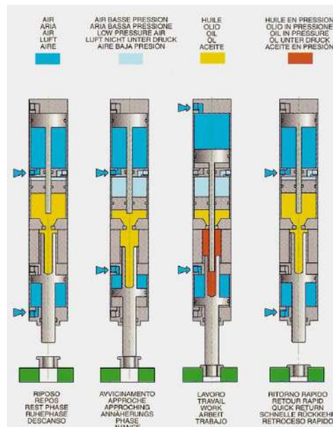
Abbildung 2 _ Betriebsprinzip
