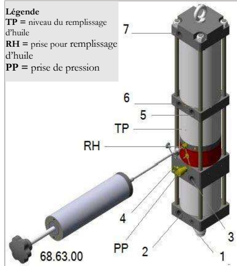
Figure 6 _ Connexion de la pompe de remplissage
