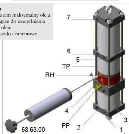
Rysunek 6 _ Podłączenie pompy do uzupełniania oleju
