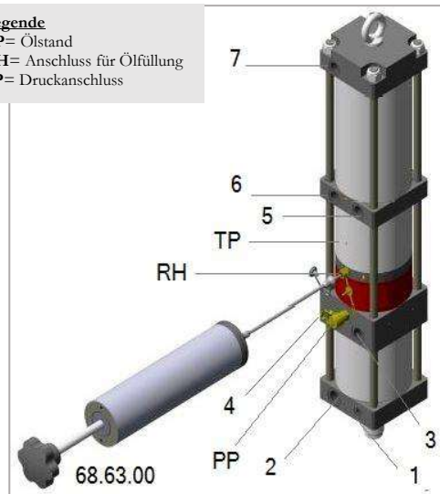
Abbildung 6 _ Anschluss der Ölladepumpe
